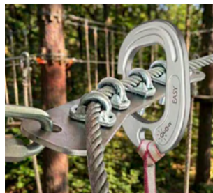
Résistant en milieu humide Toutes nos platines sont en acier inoxydable Pour câble de ligne de vie Ø 12mm ou 12,7mm
